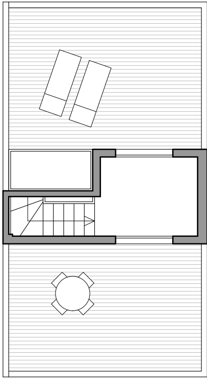
PLANTA CUBIERTA
